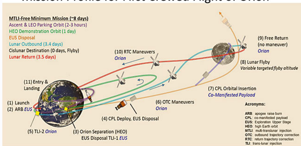
Рис. 3. На схеме, взятой из [First Crewed, 2016], Орион на обратном пути из дальнего космоса (красная траектория) сближается и выполняет стыковку с транзитным космическим кораблем на ВЭО (зеленая траектория).
